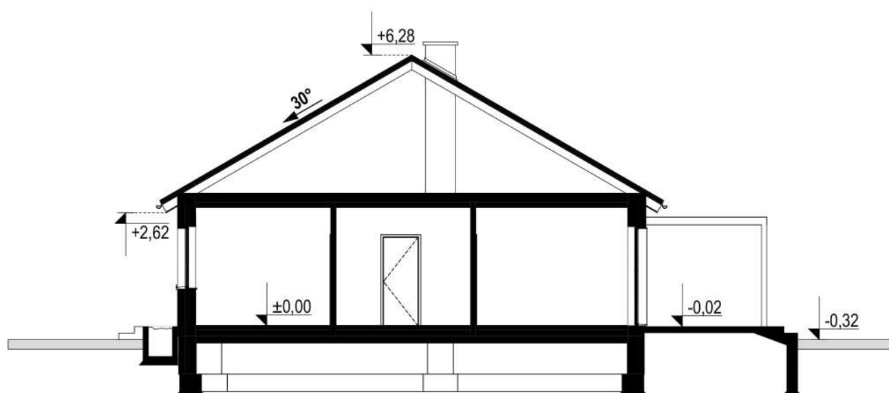
Sytuacja na działce i przekrój
