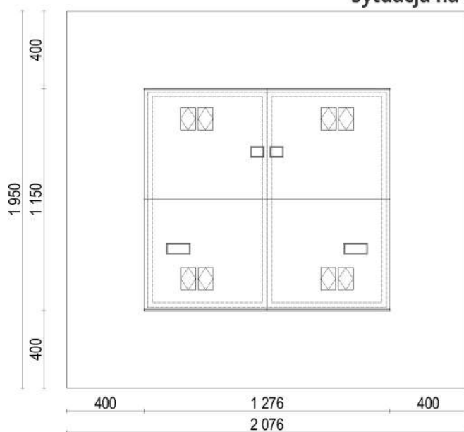
Sytuacja na działce i przekrój
